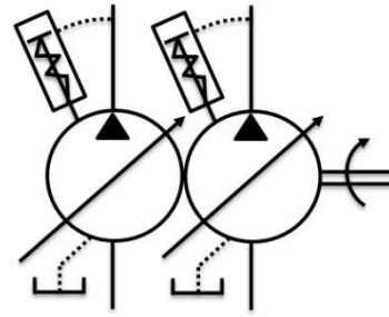
油壓記號 SYMBOL
